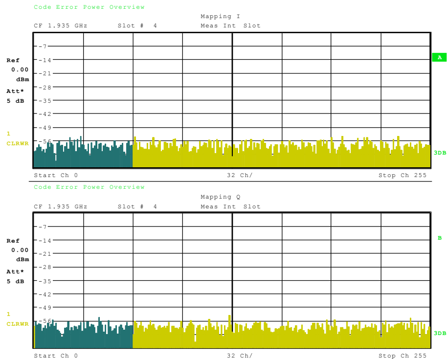
Bild 20 CDEP: Fehlerleistung ohne Codefehler
