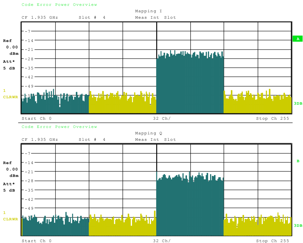
Bild 21 CDEP: Fehlerleistung eines nicht erkannten Kanals im I- und im Q Zweig
