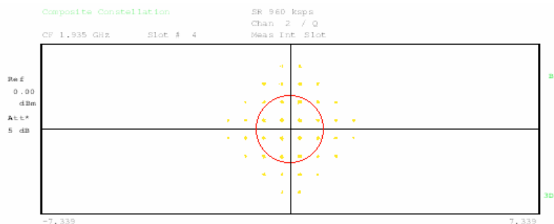
Bild16 Darstellung des Composite-Constellation-Diagramms (verwürfelte Chips)
