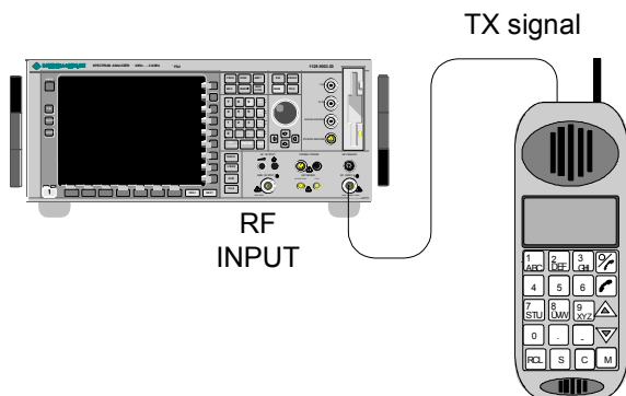
Bild 1 Mobilstations-Messaufbau
