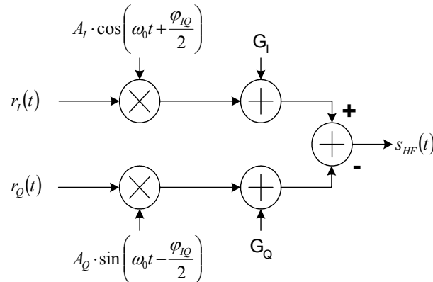
Bild 19 Grundmodell mglicher I/Q-Modulatorverzerrungen in komplexen Mixern
