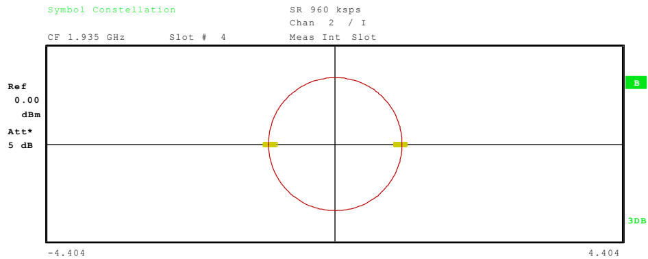
Bild 28 Symbol Constellation Diagram eines auf den I-Zweig abgebildeten Kanals
